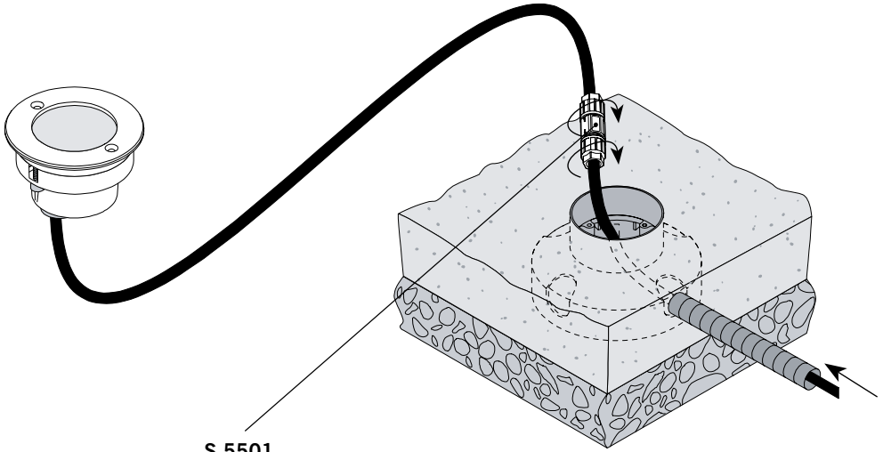
S.5501 Connettore rapido a richiesta Fast connector on request
